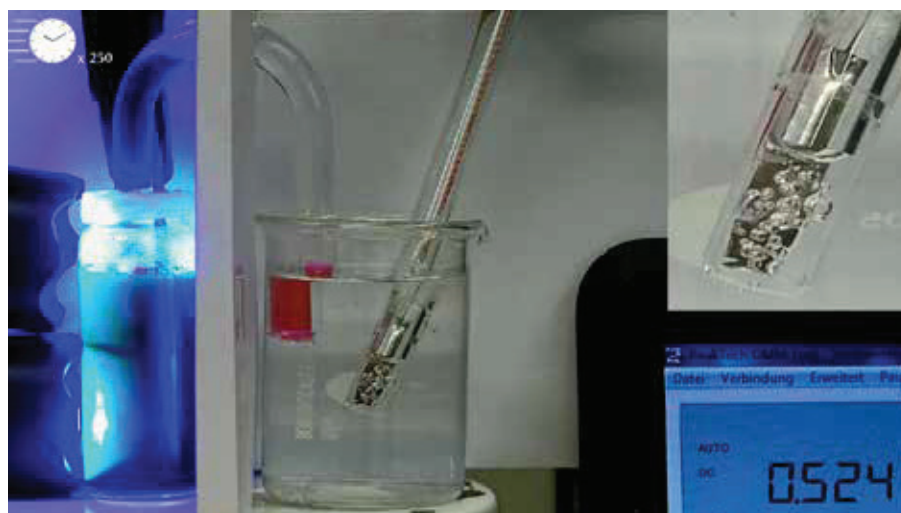
Abb. 8: Photogalvanische Zweitopfzelle zur Erzeugung von Wasserstoff
