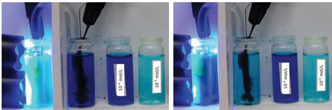
Abb. 6: Photogalvanische Zweitopfzelle zur Synthese des Reduktionsäquivalents Leukomethylenblau MBH beim Start und nach 15 min Bestrahlung
