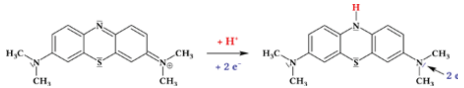
Abb. 3: Reduktion von MB + zu MBH
