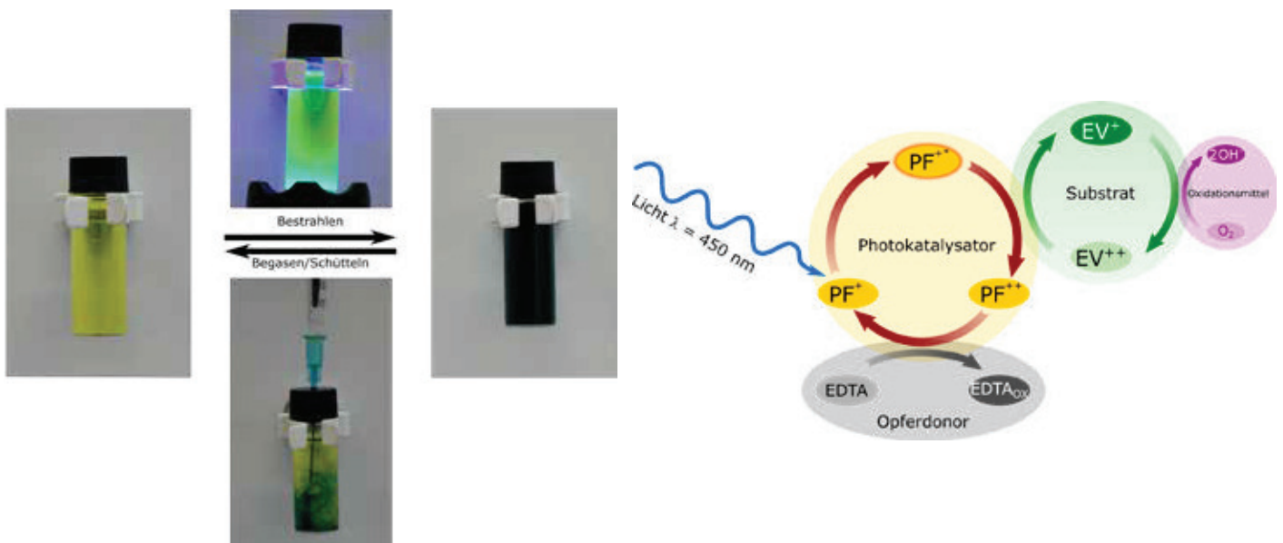
Abb. 5: Basisversion des Photo-Blue-Bottle Experiments und gekoppelte Reaktionszyklen
