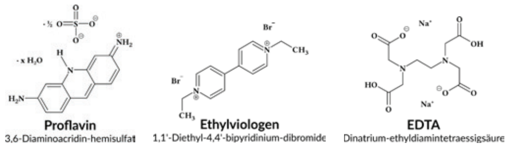
Abb. 4: Chemikalien für die Photo-Blue-Bottle Lösung
