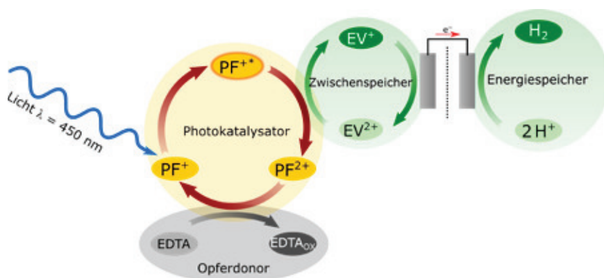
Abb. 7: Photogalvanische Zweitopfzelle zur Erzeugung von Wasserstoff
