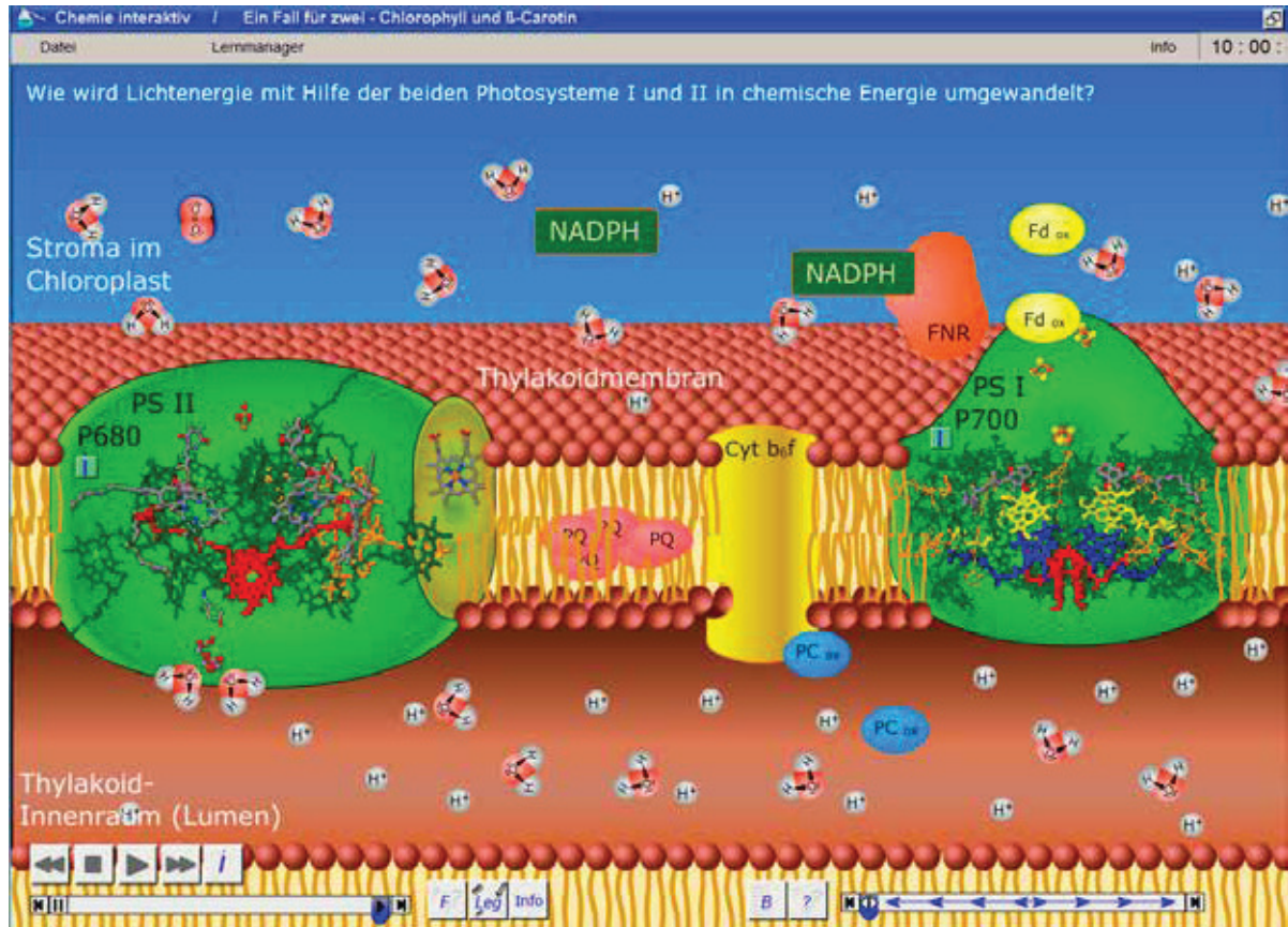
Abb. 1: Screenshot aus einer mehrteiligen Modellanimation zu den Elementarschritten bei der Lichtreaktion in Chloroplasten [1]
