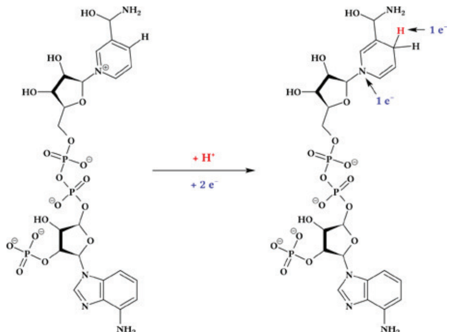
Abb. 2: Reduktion von NADP + zu NADPH
