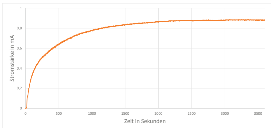
Abb. 9: Bei den photogalvanischen Zweitropfzellen wurden im photostationären Zustand annähernd konstante Stromstärken von ca. 0.9 mA gemessen
